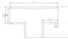
TEE
